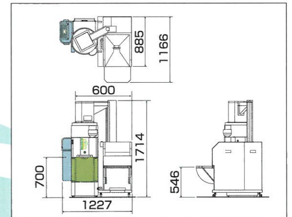
■寸法図(単位: mm)
